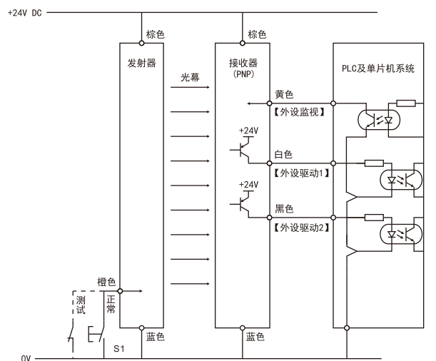
SLC系列安全光栅 (PNP) 与PLC及单片机系统接线图
