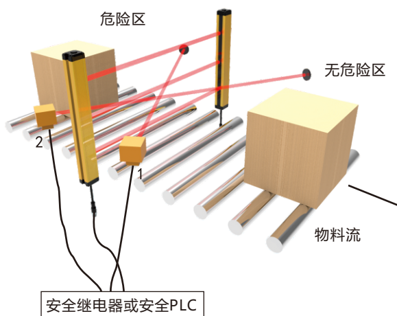
传送装置2个传感器屏蔽
