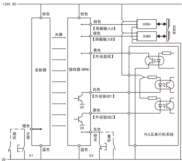
SLC-LP系安全光栅（NPN）与PLC及单片机系统接线图
