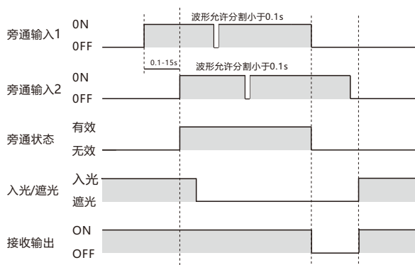
接收光栅：旁通模式时序图
