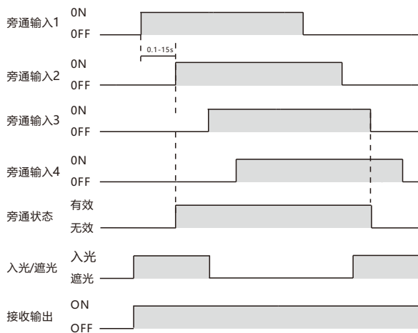
接收光栅：旁通模式时序图
